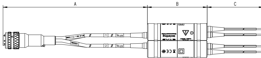
Fig. 3-1 Dimensions
